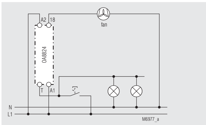
OA 8824 Time-lag circuit
