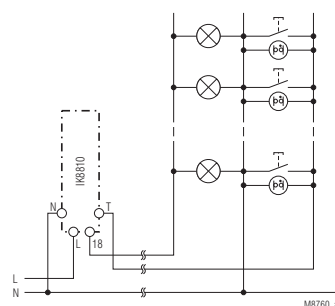
3-Leiter-Schaltung (N-getestet)
