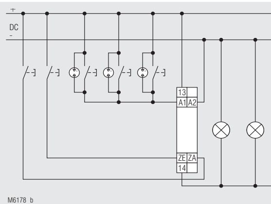
IK 8807.01 (DC activation)
