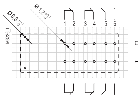
OA 5622.50/___D1 2NO / 4NC
