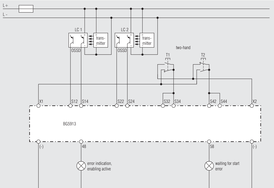
BG 5913.08/_2_ __, 2 light curtains, 1 two-hand control type IIIC (EN 574); function: 9
