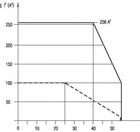
Кривая ограничения искрения при резистивной нагрузке
