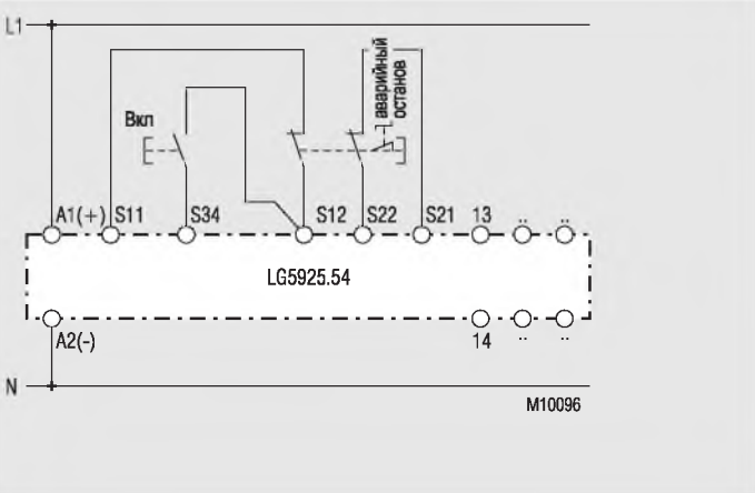
Двухканальная схема аварийного останова с контролем перекрестных замыканий.
