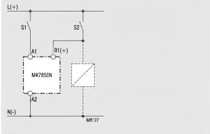
Управление с подключенной параллельной нагрузкой
