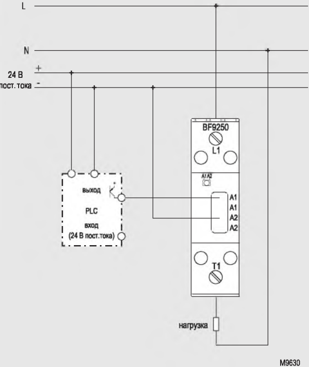
однофазная система
