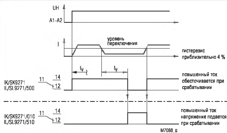
Функциональная схема IL 9271.12, SL 9271.12
