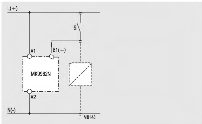
Управление с подключенной параллельной нагрузкой
