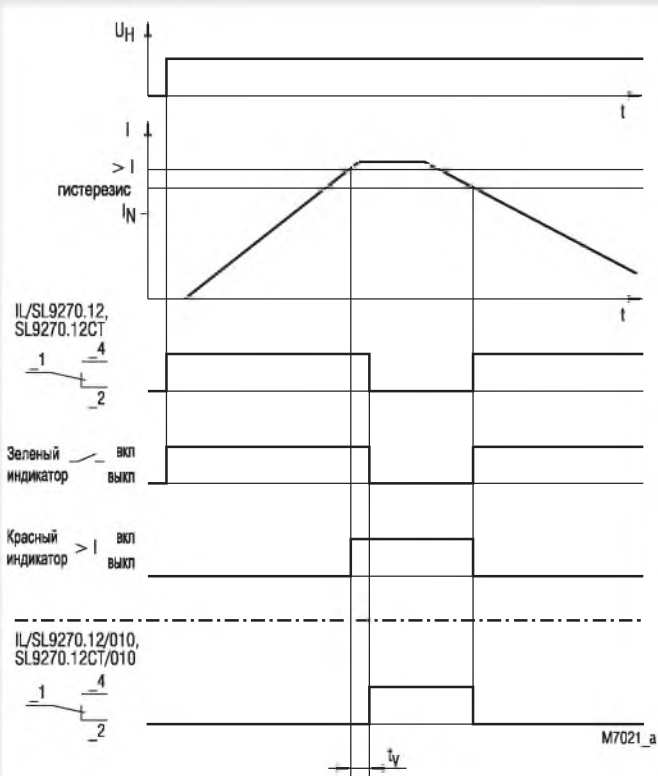
Функциональная схема IL 9270.12, SL 9270.12
