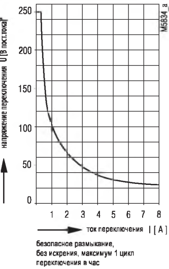
Кривая ограничения искрения при резистивной нагрузке
