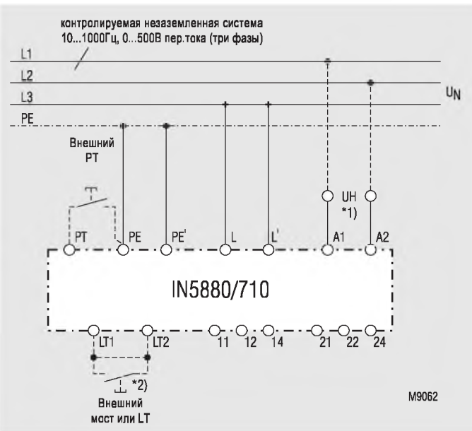
Контроль трехфазной системы питания IT
