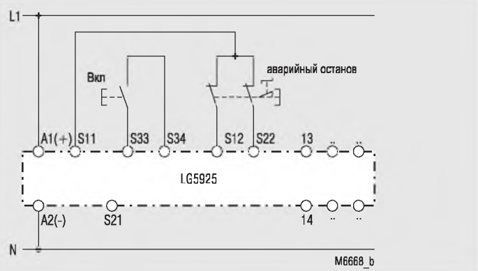
Двухканальная схема аварийного останова без контроля перекрестных замыканий.
