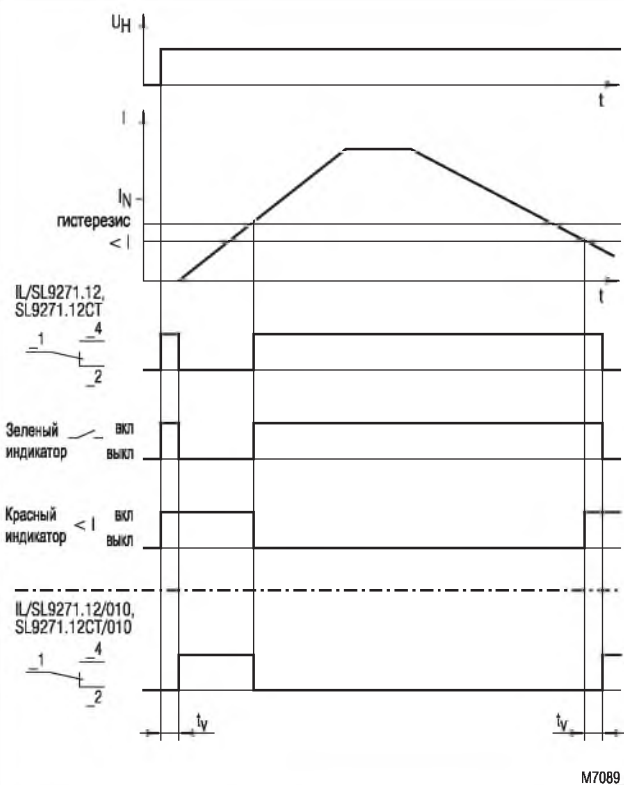
Функциональная схема IL 9271.12, SL 9271.12
