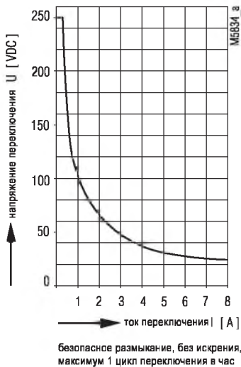
Кривая ограничения искрения при резистивной нагрузке
