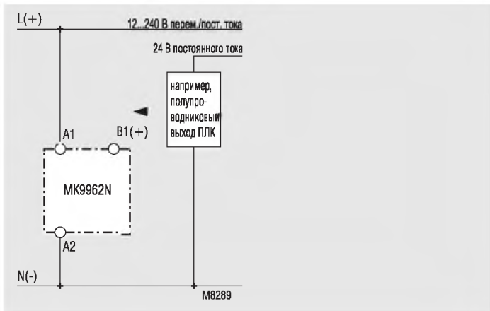
Подключение с 2 разными управляющими напряжениями
