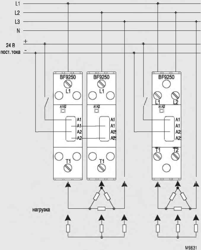
трехфазная система, управление по двум фазам
