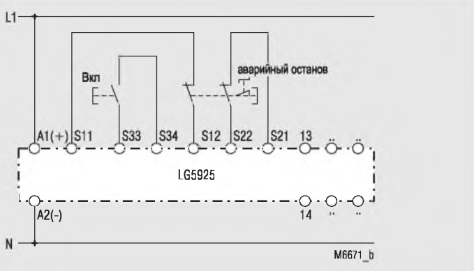
Двухканальная схема аварийного останова с контролем перекрестных замыканий.
