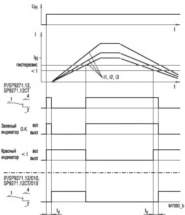
Функциональная схема IP 9271, SP 9271
