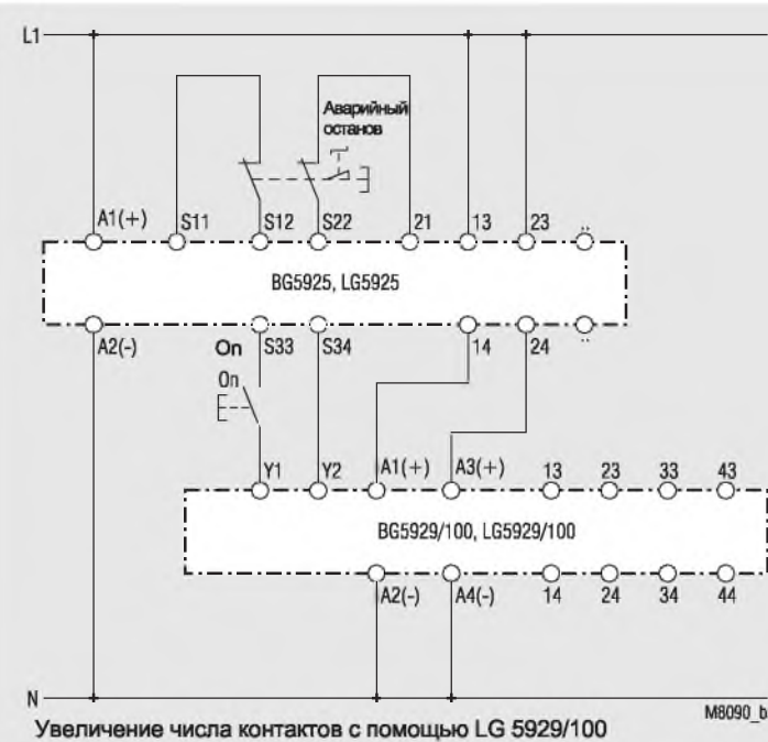
Увеличение числа контактов с помощью LG 5929/100
