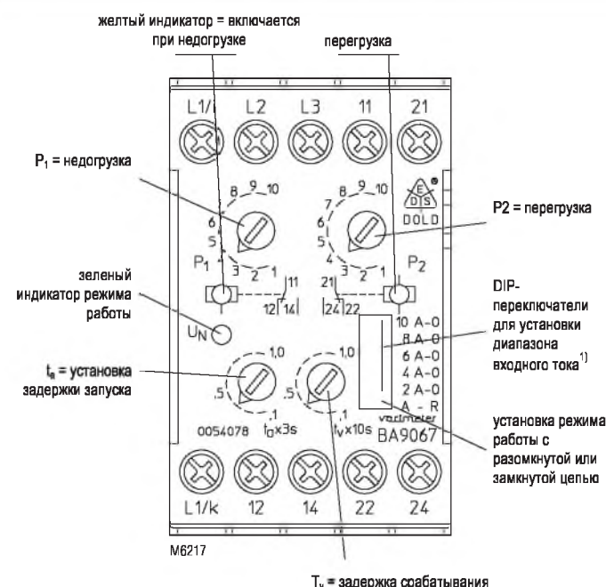
BA 9067.38 для тока > 10 А с трансформатором тока
