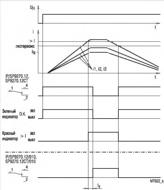
Функциональная схема IP 9270, SP 9270
