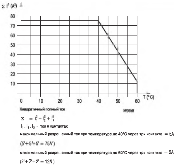
Кривая ухудшения токов защищенных контактов
