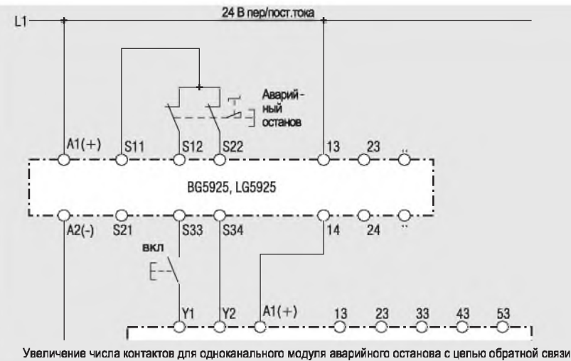
Увеличение числа контактов для одноканального модуля аварийного останова с цепью обратной связи
