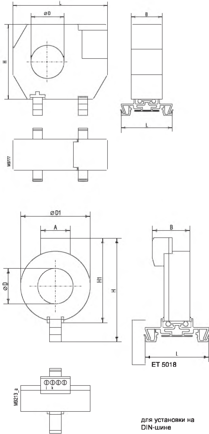
Трансформатор дифференциальных токов ND 5018/030
