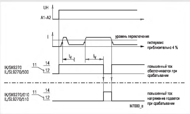
Функциональная схема IL 9270.12, SL 9270.12
