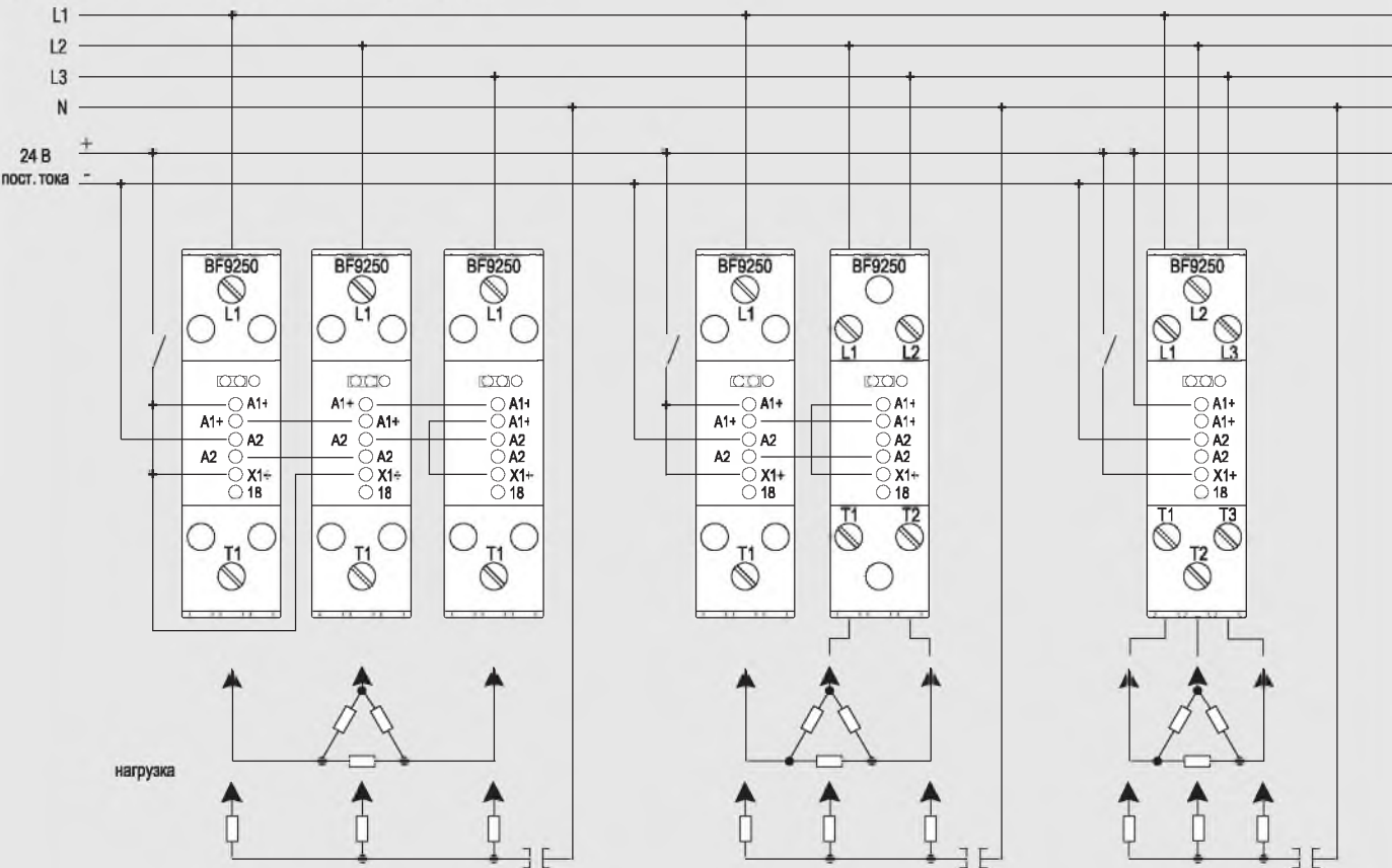
Трехфазная нагрузка, переключаемая тремя однополюсными полупроводниковыми контакторами
