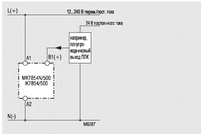
Подключение с 2 разными управляющими напряжениями
