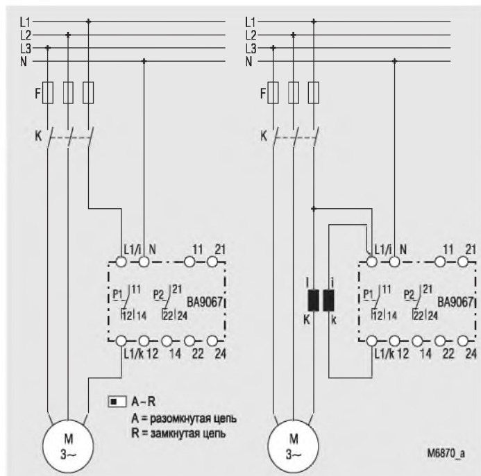
BA 9067.38 для тока < 10 А
