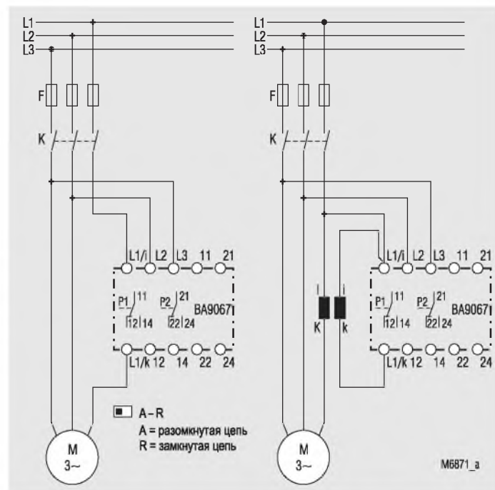
BA 9067.38/001 для тока < 10 А
