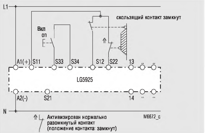
Двухканальный контроль предохранительных ворот.
