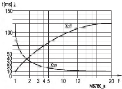
Задержка переключения
